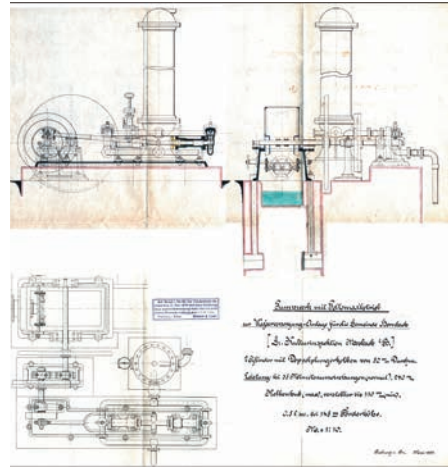
Der Plan des Stürzenhardter Pumpwerks von 1899. (Stadtarchiv Buchen)
